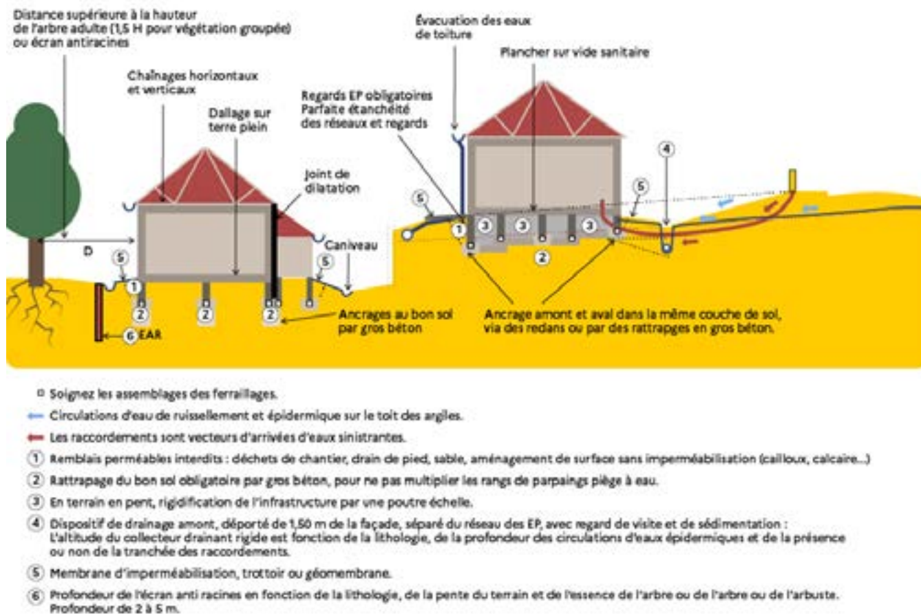
Figure 9 : Synthèse des mesures de prévention et d'adaptation du bâti au phénomène RGA (guide CSTB, 2021)
